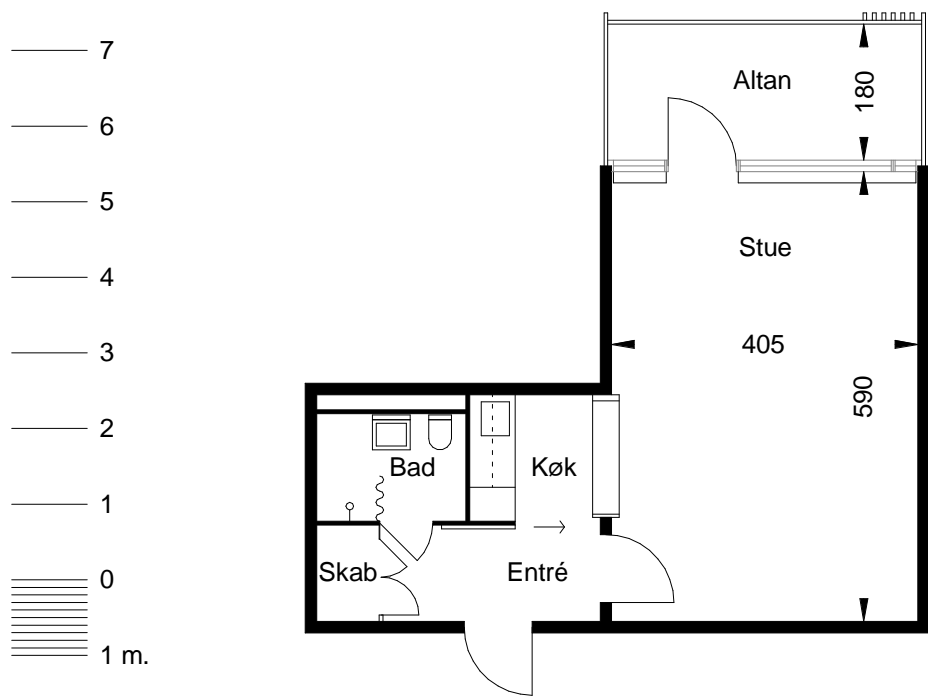
Type D 1 værelse 1:100 Seniorboliger Lions Park Hillerød
