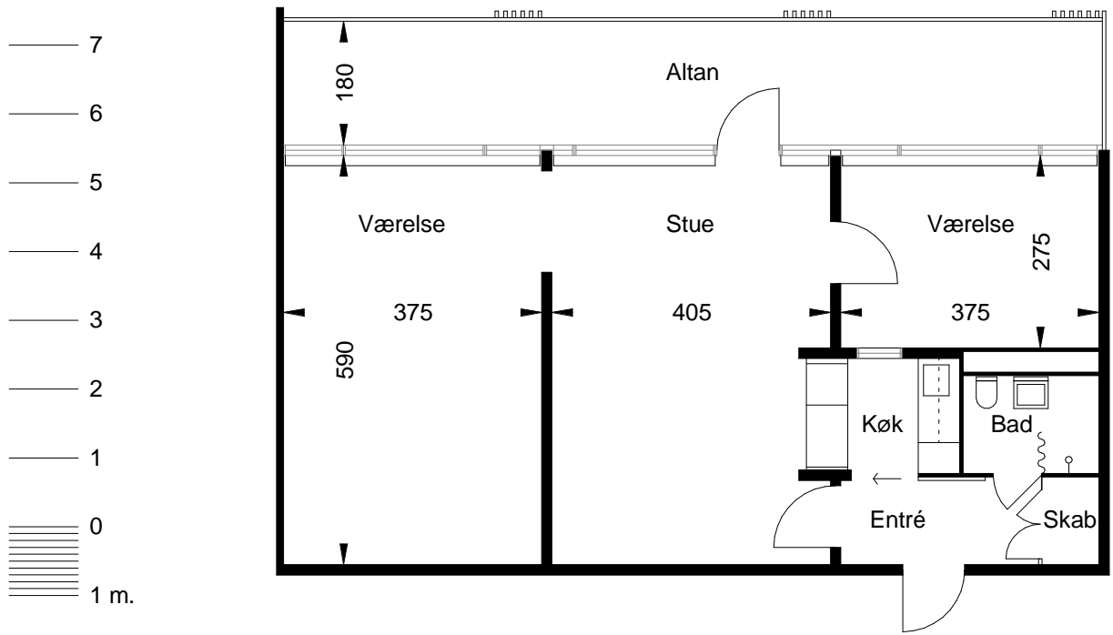
Type A 3 værelser 1:100 Seniorboliger Lions Park Hillerød
